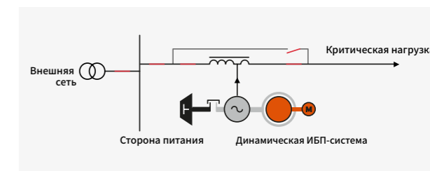
Статический ИБП
