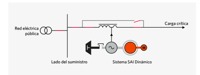
SAI dinámico
