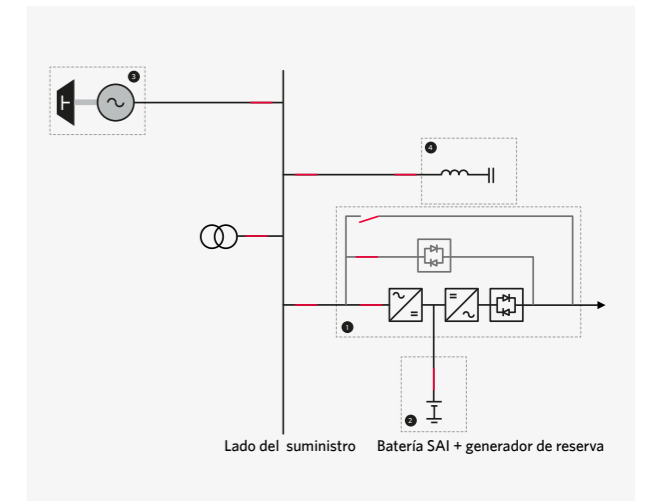
SAI estático
