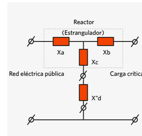
Diagrama eléctrico equivalente del filtro activo
