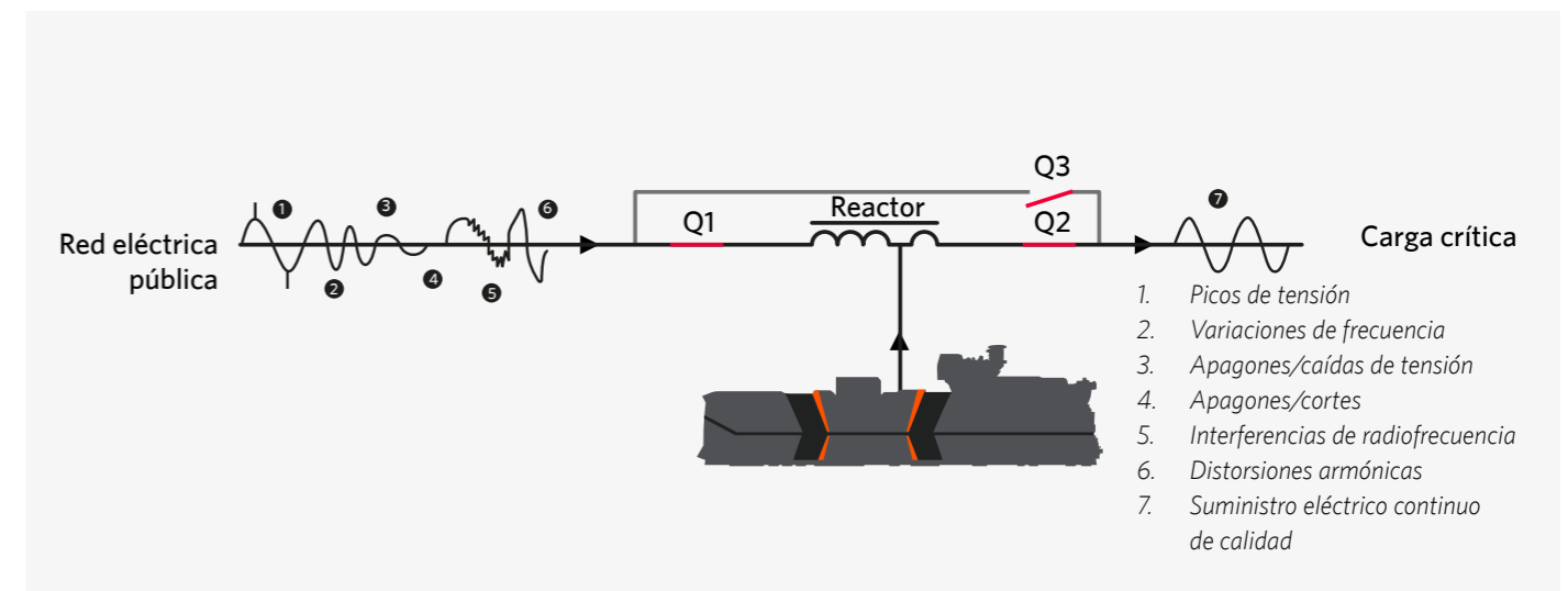
Una solución de SAI dinámico actúa como un filtro para todo tipo de perturbaciones en la red pública.
