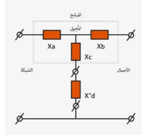
رسم بياني للمرشح النشط
